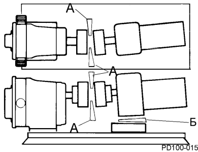
Малюнок 19 - Перевірка кутового вирівнювання
