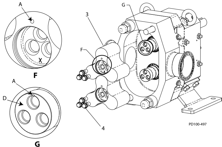
Малюнок 56 - Установка ротора
