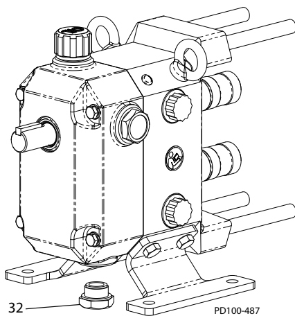
Малюнок 37 - зніміть пробку для зливання мастила
