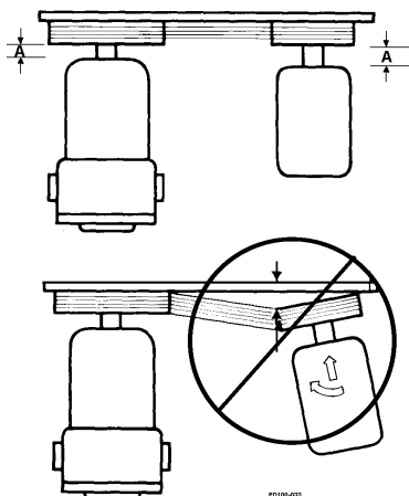
Малюнок 21 - Перевірка вирівнювання ремінної і ланцюгової передачі
