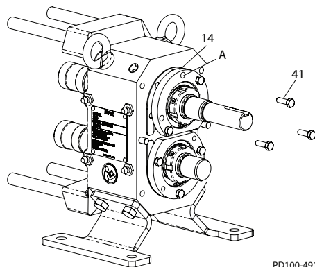
Малюнок 40 - Дістаньте гвинти
