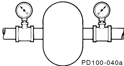
Малюнок 17 - Датчики тиску і вакуумні манометри
