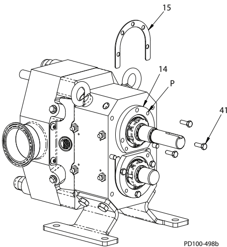
Малюнок 58 - Установіть шайби
