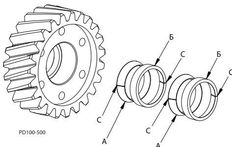
Малюнок 60 - Установка блокувального елемента
