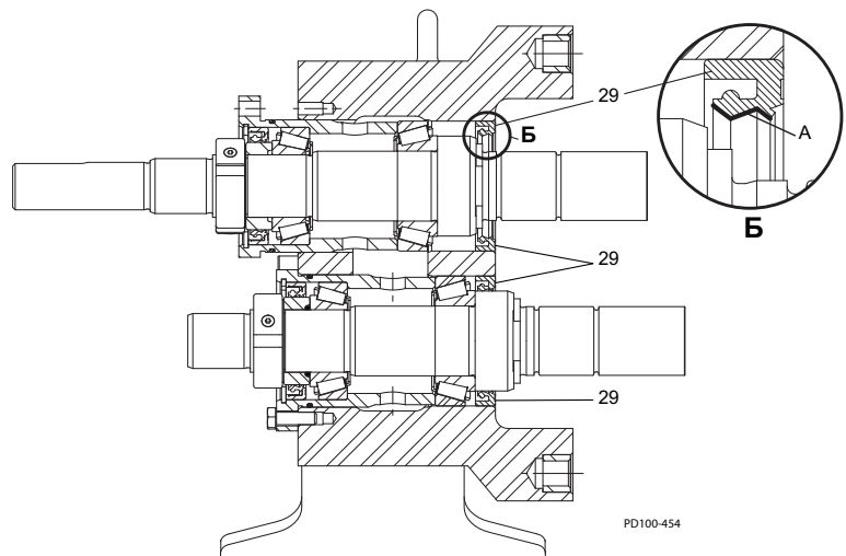
Малюнок 48 - нанесіть підшипникове мастило
