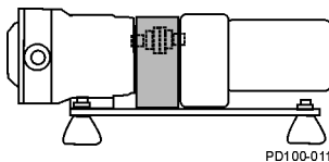
Малюнок 6 - Вирівнювальні і/або віброізоляційні опори
