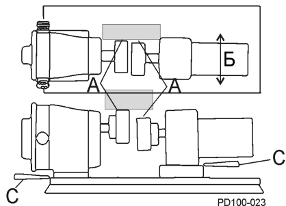
Малюнок 20 - Перевірка вирівнювання для забезпечення паралельності
