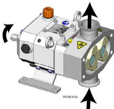
Малюнок 25 - Pump Rotation
