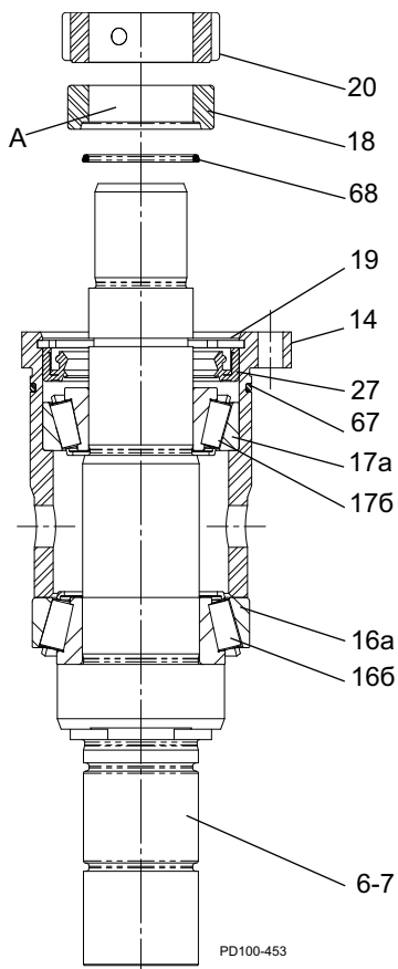
Малюнок 47 - Підшипник в зборі
