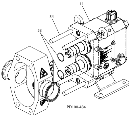
Малюнок 33 - Демонтаж корпусу насоса
