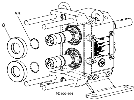
Малюнок 52 - Установка ущільнення вала
