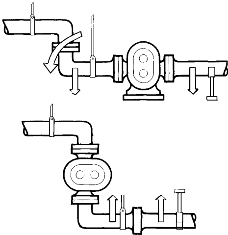
Малюнок 8 - Опора трубопроводу
