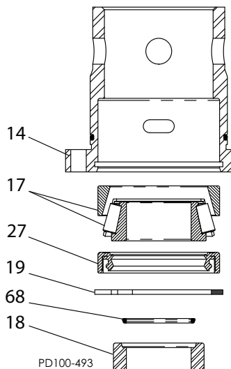
Малюнок 43 - Зніміть задній підшипник з валу.
