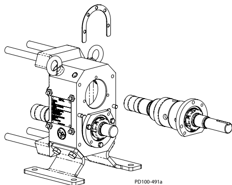
Малюнок 41 - Зніміть вал
