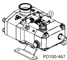
Малюнок 3 - Встановлений збоку, з лівої сторони (вид з кришки насоса)
