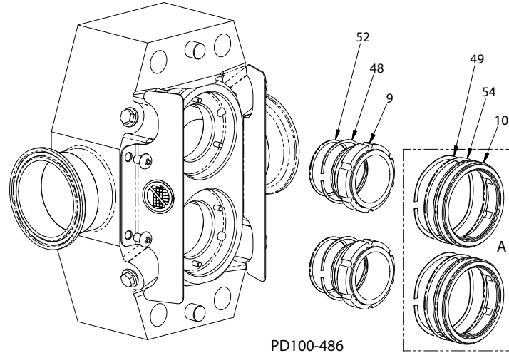
Малюнок 35 - Зніміть ущільнення
