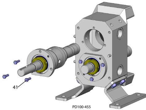
Малюнок 49 - Зафіксуйте кріпінними гвинтами
