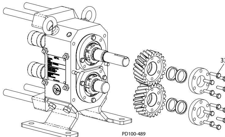
Малюнок 39 - Зніміть редуктор і замковий вузол
