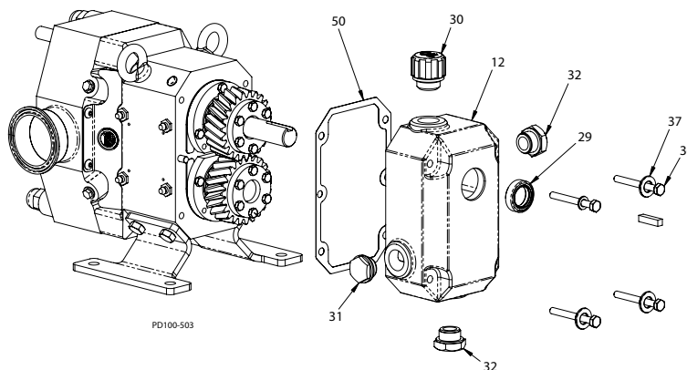
Малюнок 65 - Установка кришки редуктора
