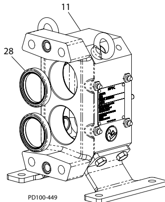
Малюнок 44 - Установка передніх ущільнень
