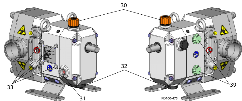
Малюнок 26 - Точки змащування
