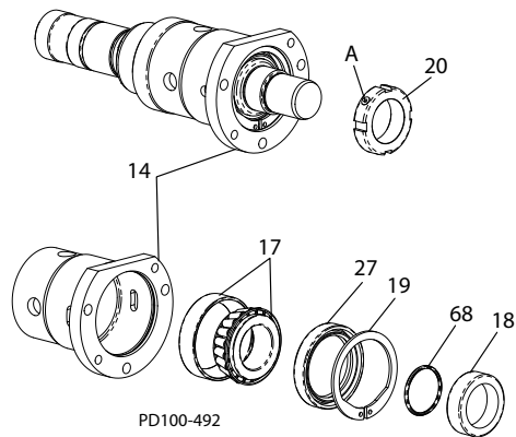
Малюнок 42 - Зніміть підшипник
