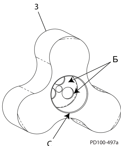
Малюнок 55 - Ротор
