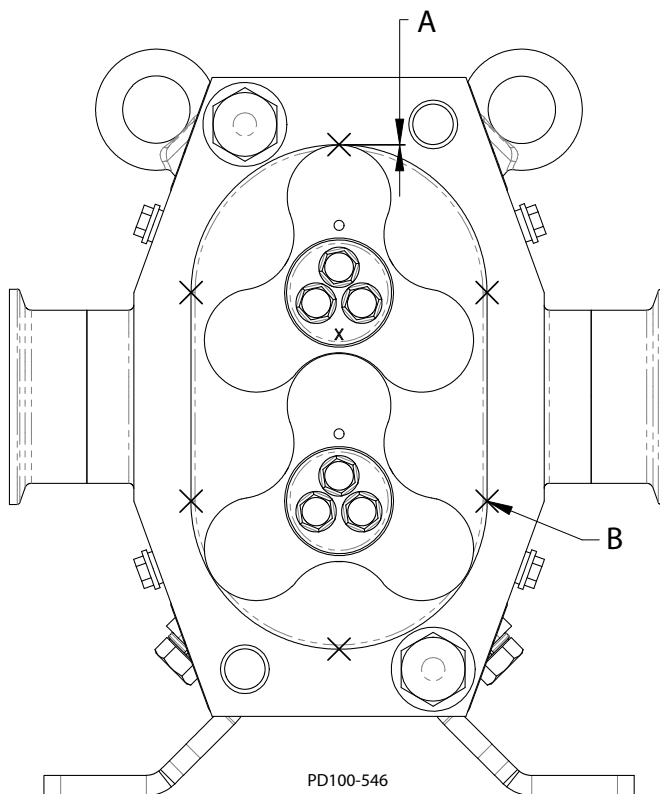
Малюнок 64 - Перевірка радіального зазору
