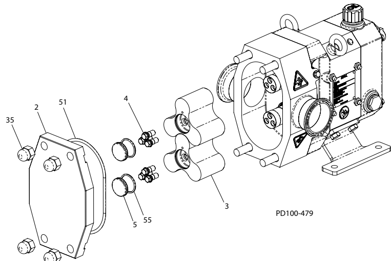
Малюнок 30 - Зняття кришки насоса і ротора
