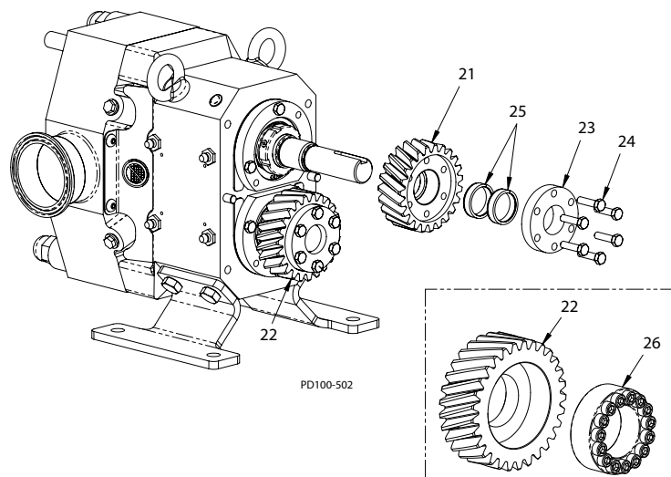
Малюнок 61 - Установка зубчастих передач
