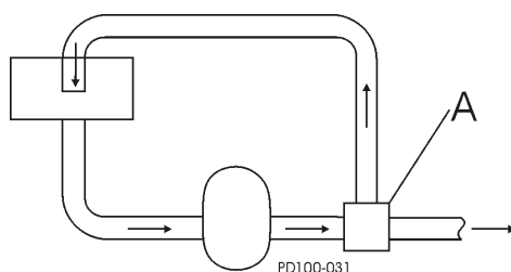
Малюнок 15 - Клапани скидання тиску
