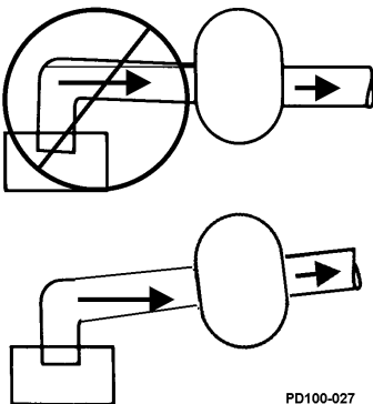
Малюнок 11 - Вирівняйте трубопровід, щоб уникнути появи повітряних пробок при всмоктуванні повітря
