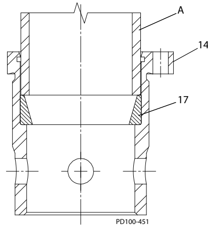
Малюнок 46 - Установіть зовнішнє кільце заднього підшипника
